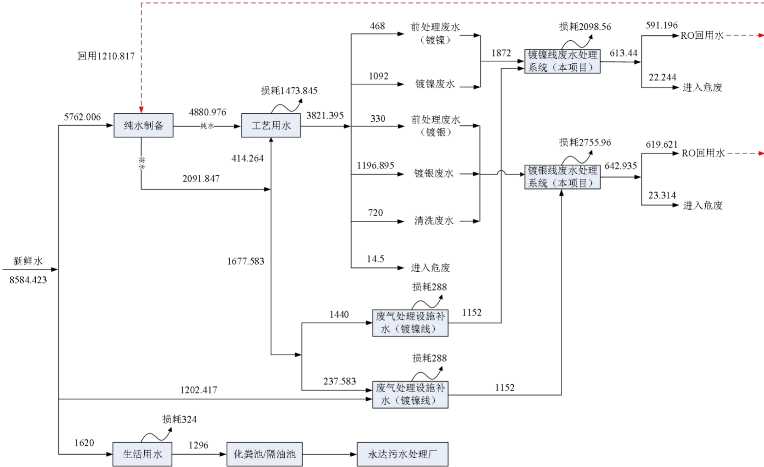
图 3.2.9-1 本项目用排水平衡图 (t/a)
