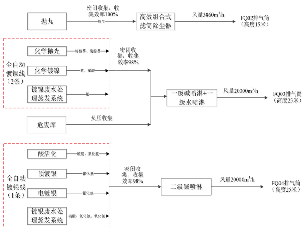
图 6.1-1 本项目废气收集处理流程图
