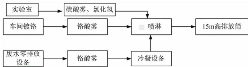
图 3.1-2 现有项目废气处理路径示意图
