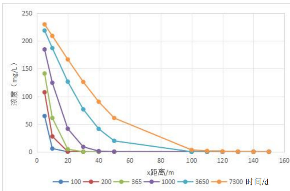
图 5.2-2 含水层中氰化物运移情况示意图
