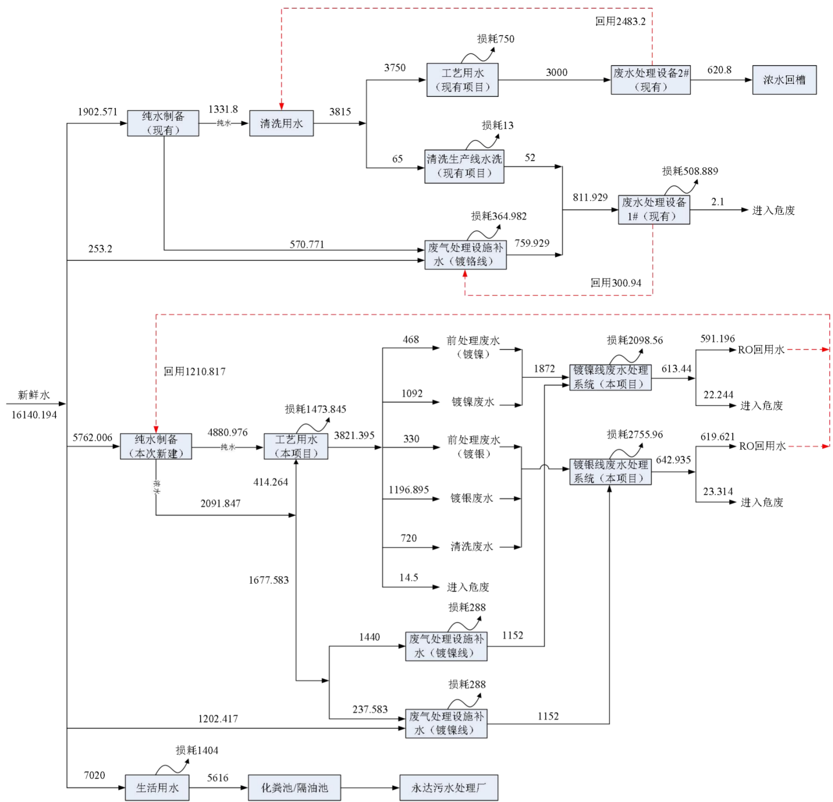
图 3.2.9-2 本项目建成后全厂用排水平衡图 (t/a)
