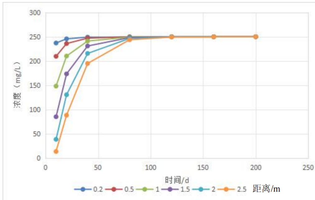
图 5.2-3 土壤环境影响预测结果图
