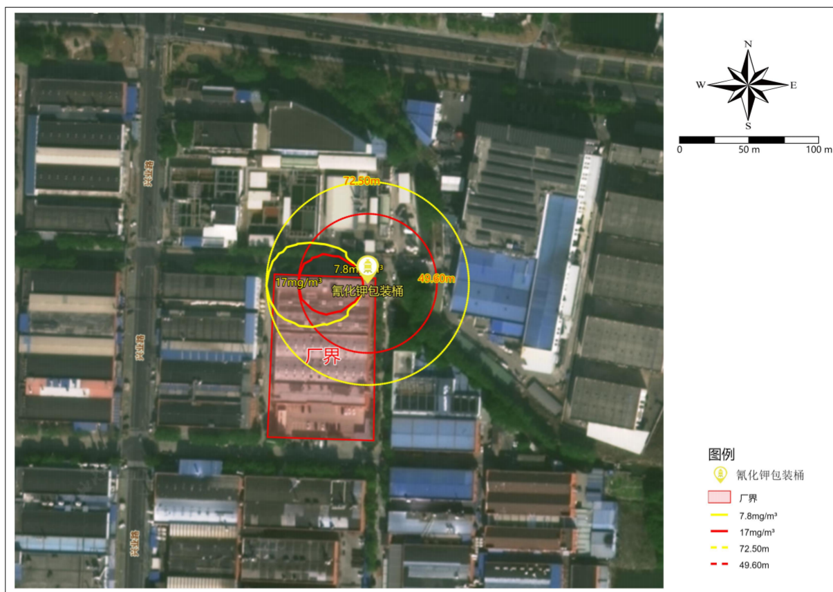
图 5.2-5 氰化钾受潮释放氰化氢泄漏预测浓度达到毒性终点浓度的最大影响范围图
