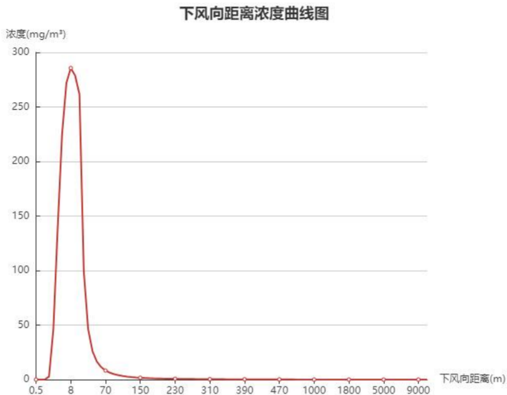
图 5.2-4 氰化钾受潮释放氰化氢泄漏风险事故下风向距离浓度曲线图
