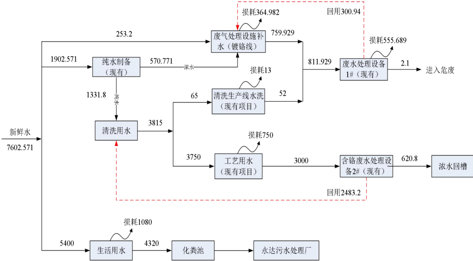
图 3.1-3 现有项目用排水平衡图 (t/a)
