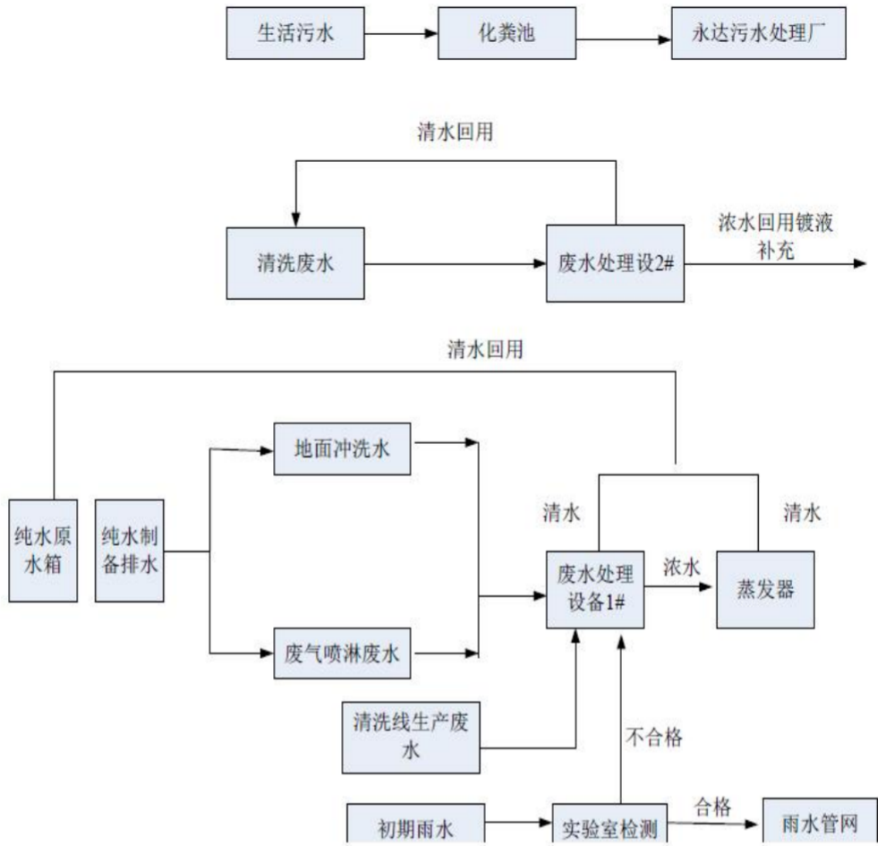
图 3.1-3 厂区废水流向示意图
